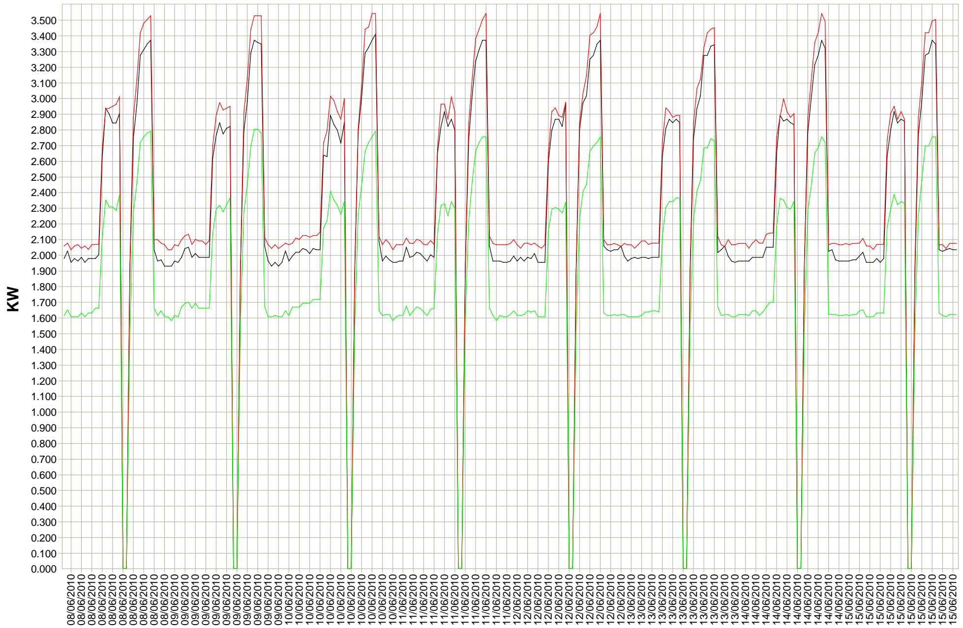
Armoire 5770 Puissance Réelle R S T 08/06/2010 - 15/06/2010
